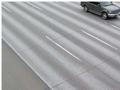
Longitudinal Cracking
